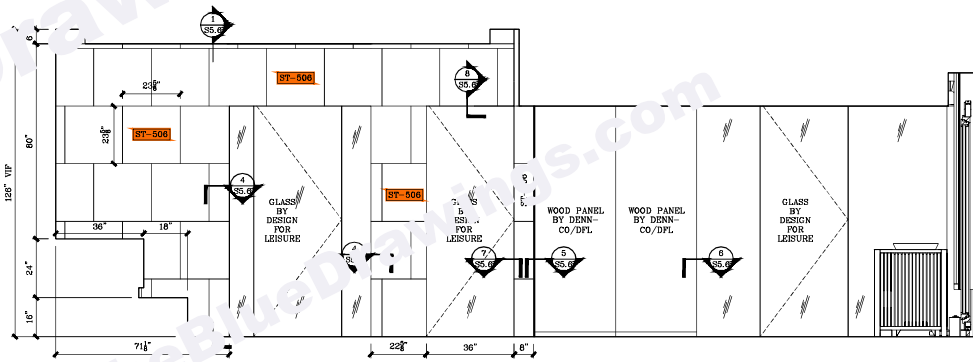
C ELEVATION SCALE: 1/2"=1'-0"
