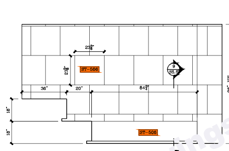
Y ELEVATION SCALE: 1/2"=1'-0"
