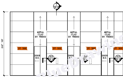
S ELEVATION SCALE: 1/4"=1'-0"
