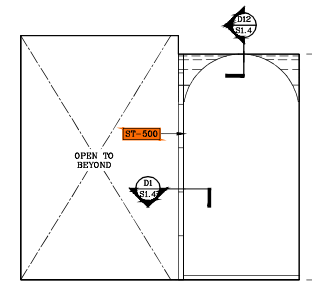
L ELEVATION SCALE: 1/4"=1'-0"
