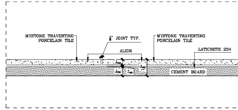
D15 VERTICAL DETAIL SCALE: 6"=1'-0"
