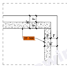
④ PLAN DETAIL SCALE: 6"=1'-0"
