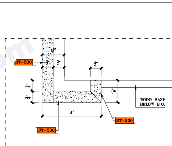
① PLAN DETAIL SCALE: 6"=1'-0"
