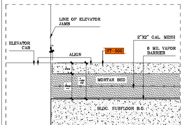
⑦ VERTICAL DETAIL SCALE: 6"=1'-0"
