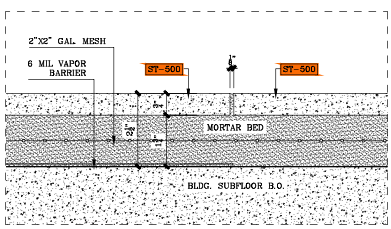
⑥ VERTICAL DETAIL SCALE: 6"=1'-0"
