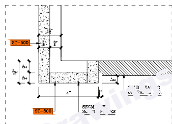
⑫ VERTICAL DETAIL SCALE: 6"=1'-0"
