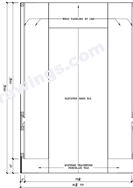
C ELEVATION SCALE: 1"=1'-0"
