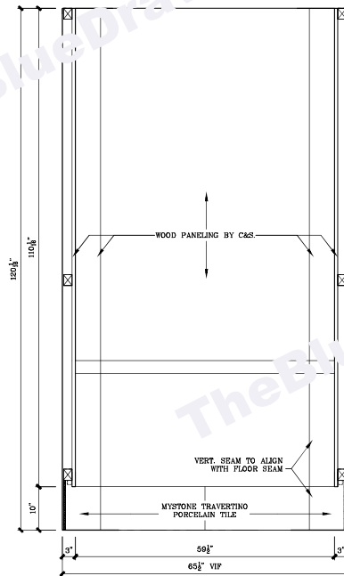
B ELEVATION SCALE: 1"=1'-0"
