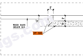
⑤ PLAN DETAIL SCALE: 6"=1'-0"
