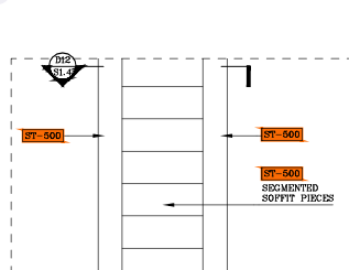
⑪ REPL. CLG. PLAN PORTAL SCALE: 6"=1'-0"
