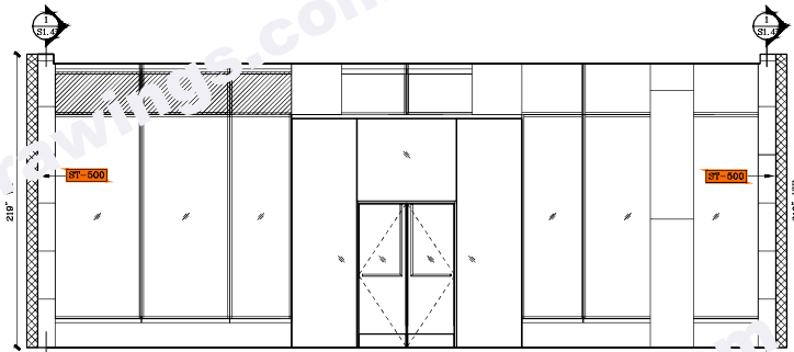
B ELEVATION SCALE: 1/4"=1'-0"
