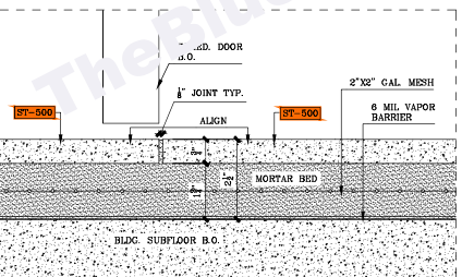
⑨ VERTICAL DETAIL SCALE: 6"=1'-0"
