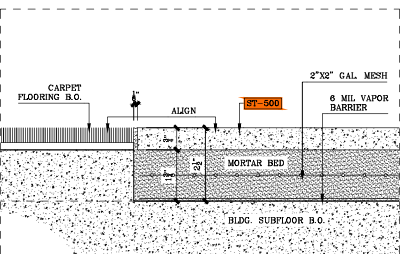
⑧ VERTICAL DETAIL SCALE: 6"=1'-0"
