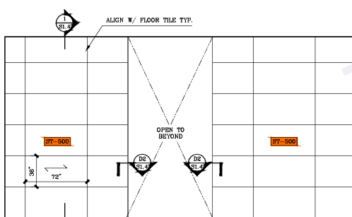
P ELEVATION SCALE: 1/4"=1'-0"
