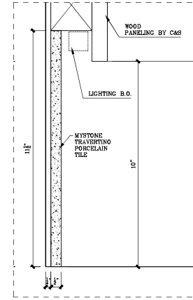
D16 VERTICAL DETAIL SCALE: 6"=1'-0"
